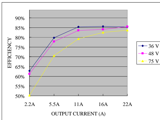
Vo=1.5 V
