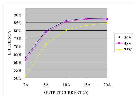
Vo=1.8 V
